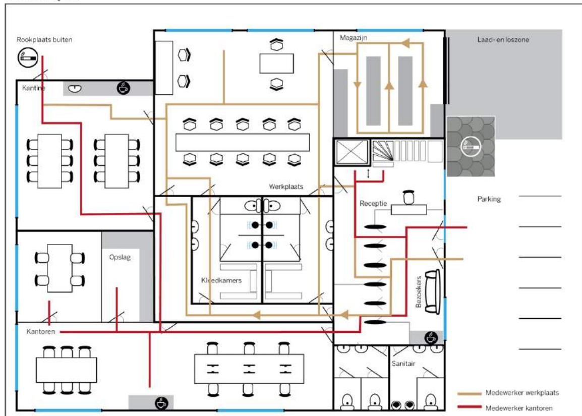
Figuur 10. Circulatieplan
